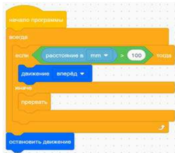
Рис. 31. Пример программы
